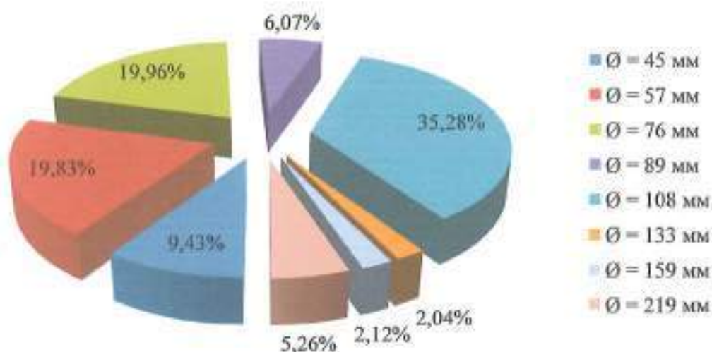
Рисунок 2.3.2.2 – Доли протяженности участков трубопроводов тепловых сетей котельных ООО УК "Егорьевское" различных диаметров
