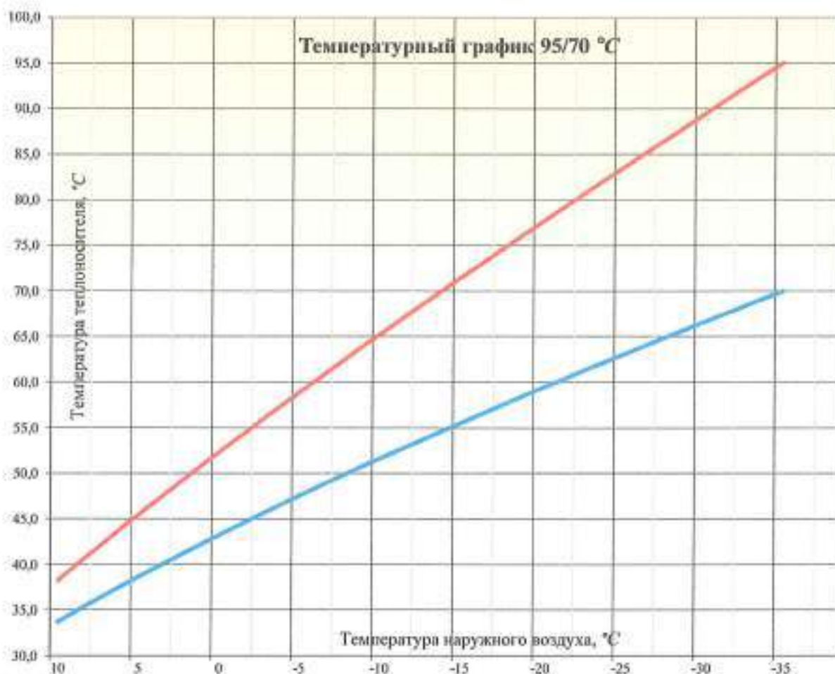
Рисунок 2.3.4.1 – График регулирования отпуска тепла
